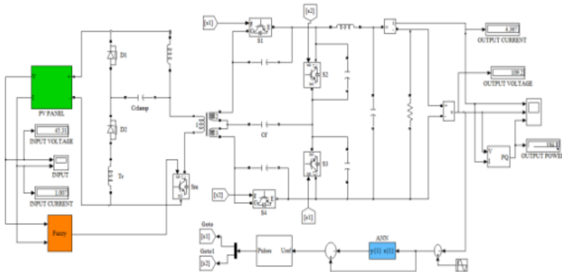
Fig.3.Output Simulink
